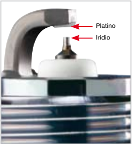
Elettrodo centrale con riporto in lega all'Iridio ed elettrodo di massa con riporto in lega al Platino, entrambi saldati al laser: accensioni sicure e il massimo della resistenza per tutta la durata di esercizio.
